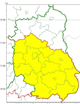
Opady marznące 2024-12-27 13:05
